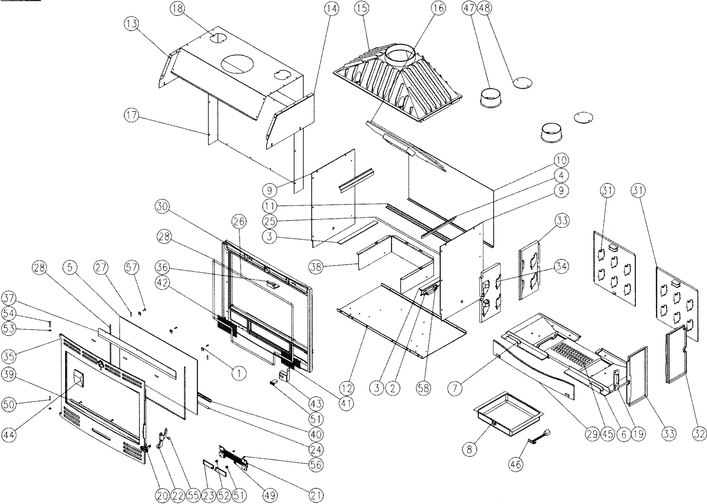
Eclaté 3283
