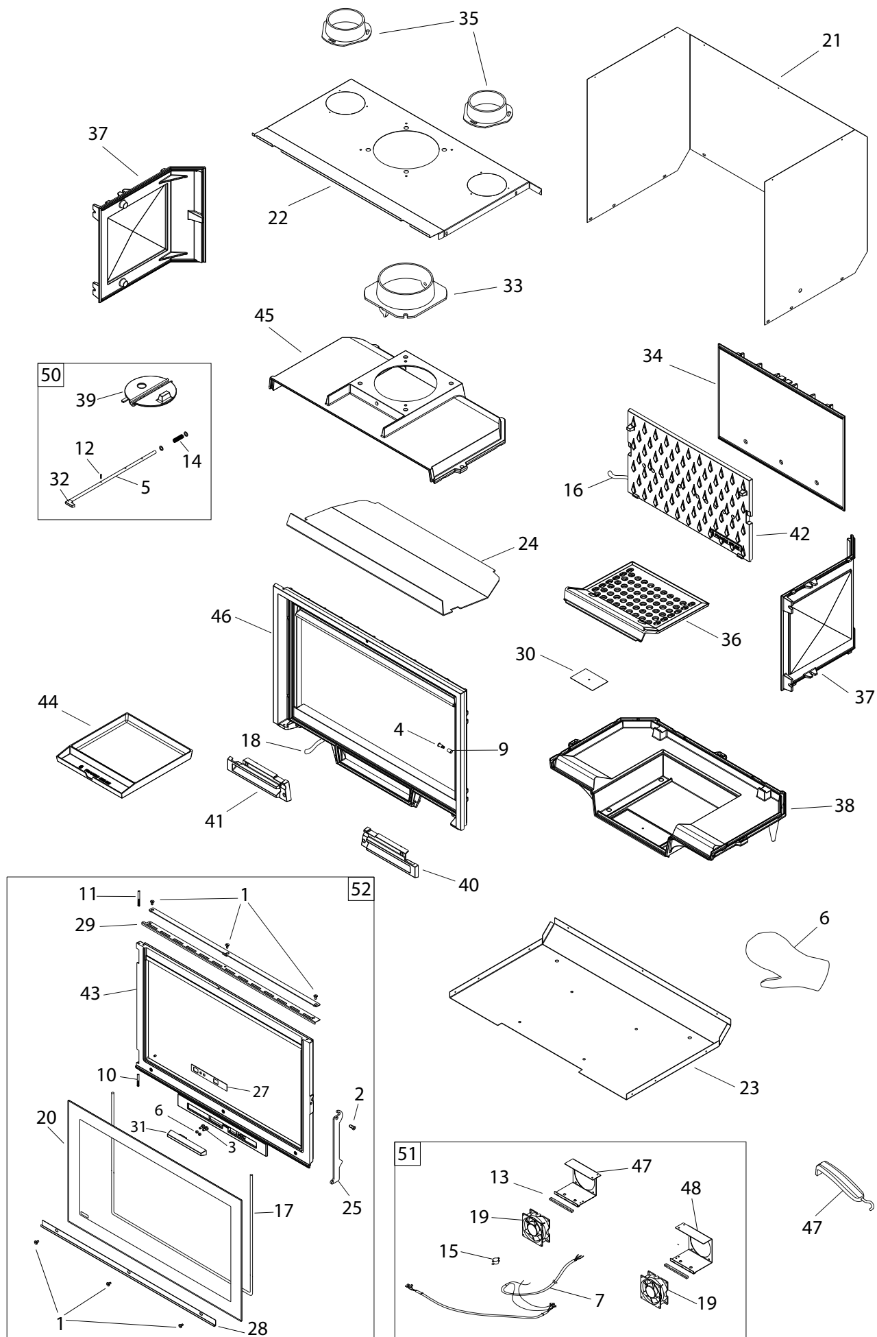
Figure 19 - Vue éclatée
