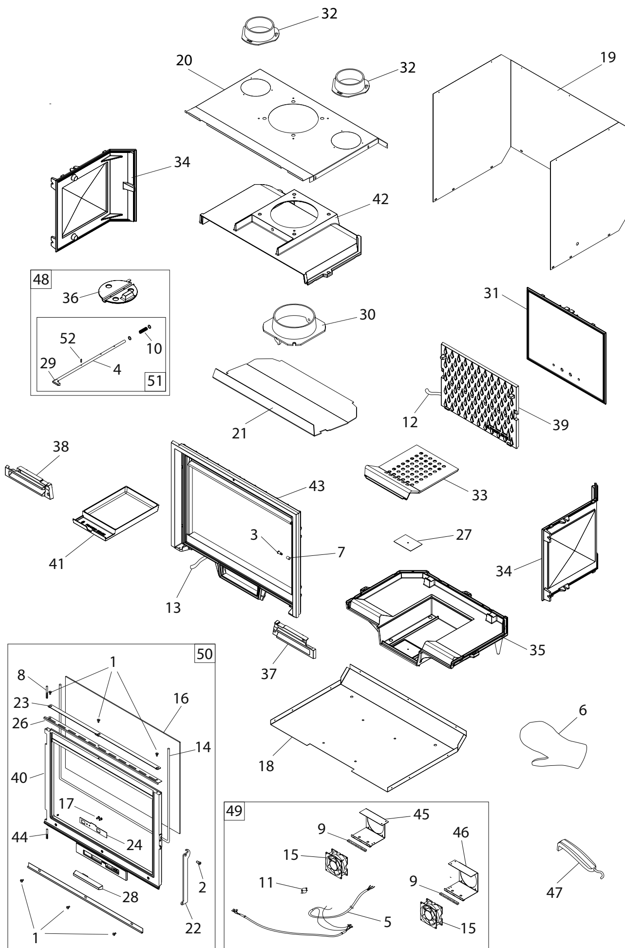
Figure 19 - Vue éclatée
