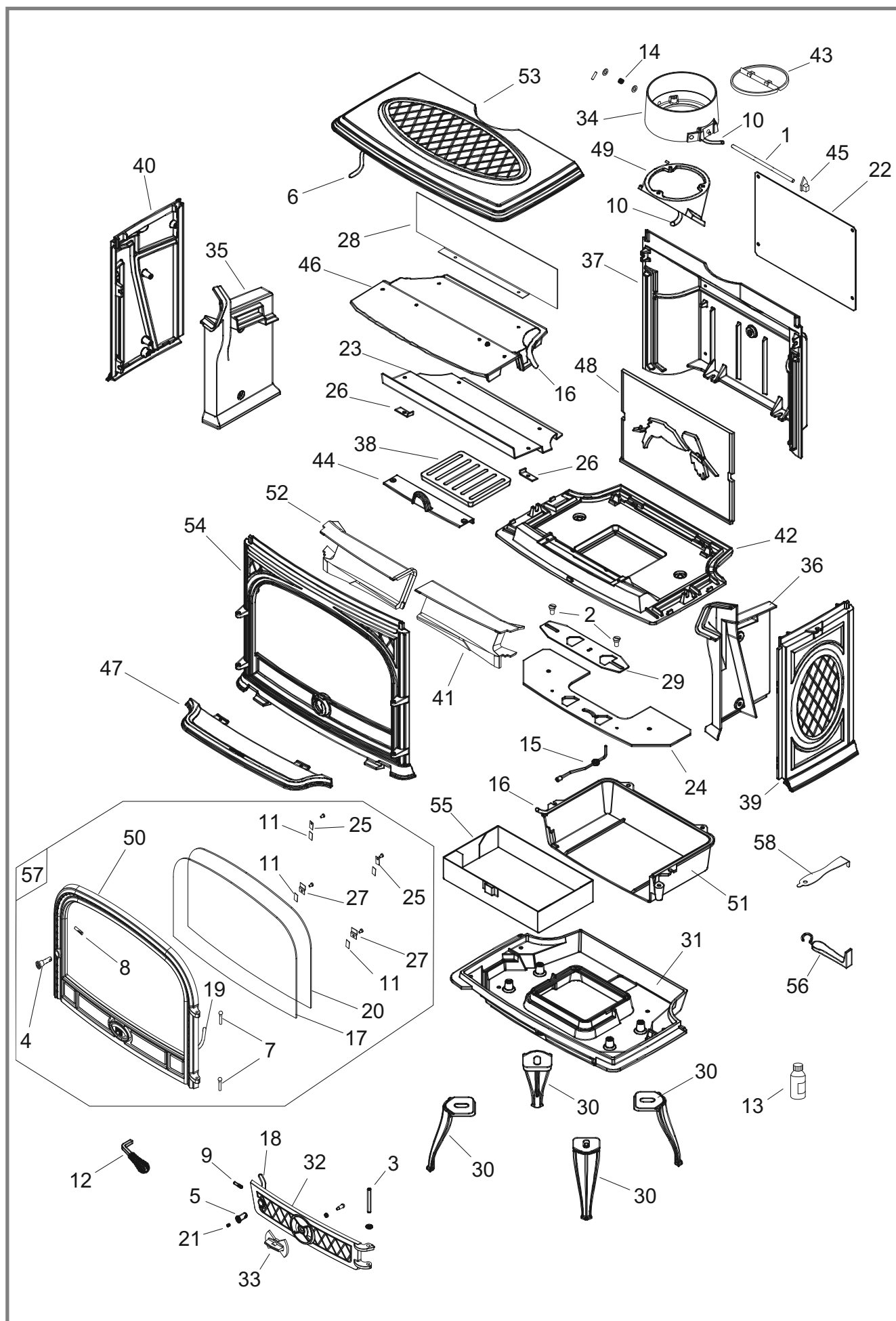
Figure 7 - Vue éclatée de l'appareil
