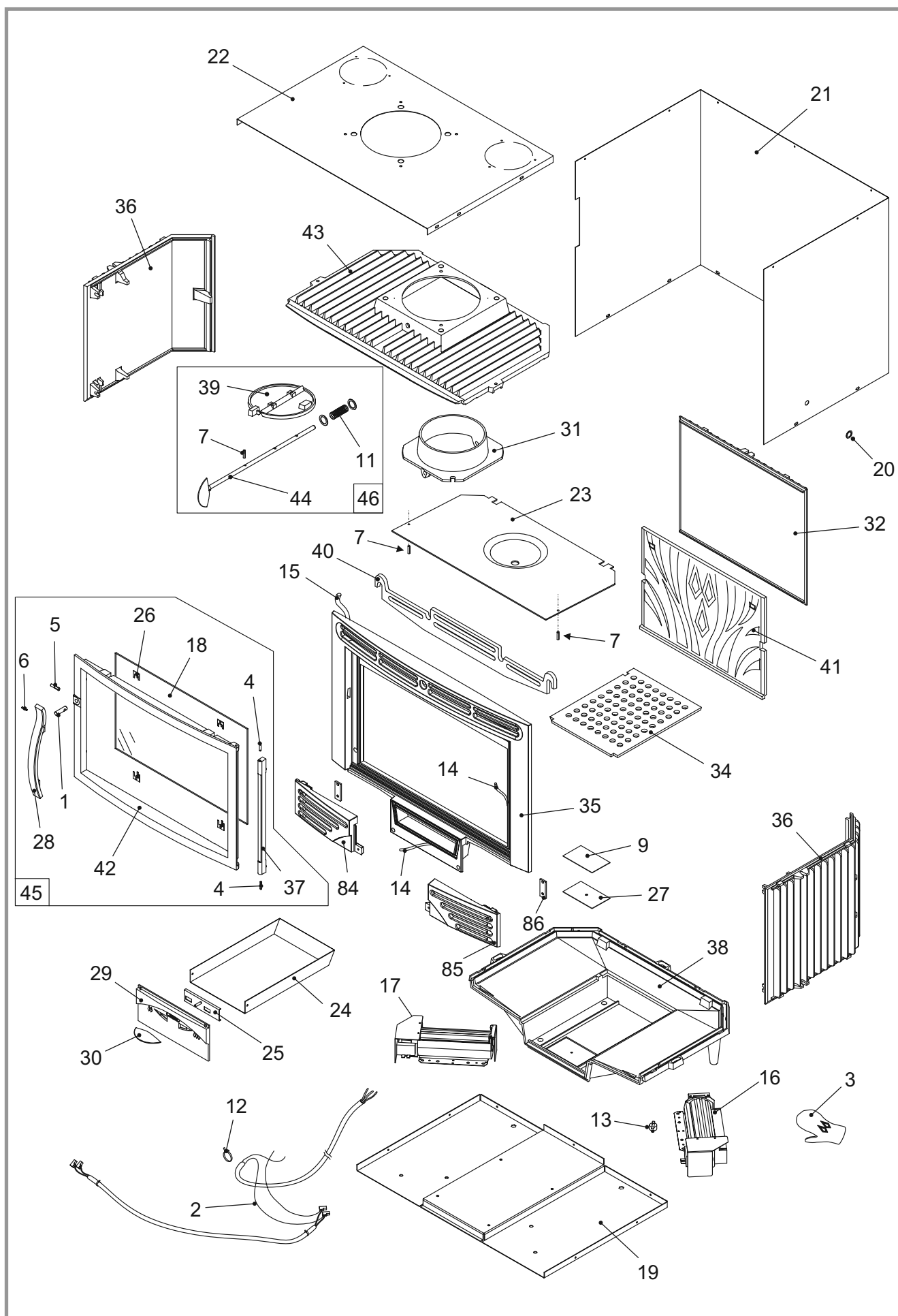
Figure 13 - Vue éclatée de l'appareil 134 10 20 Y
